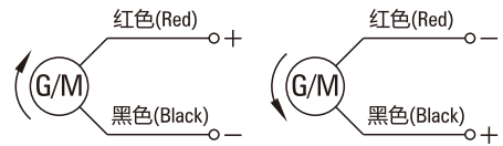
电机接线图 Wiring Diagram
